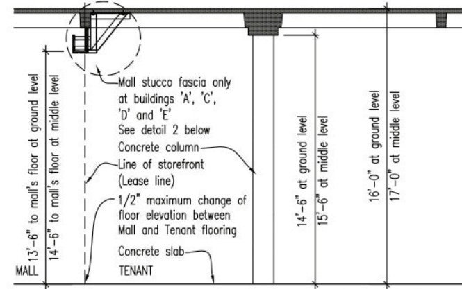
Longitudinal Section
