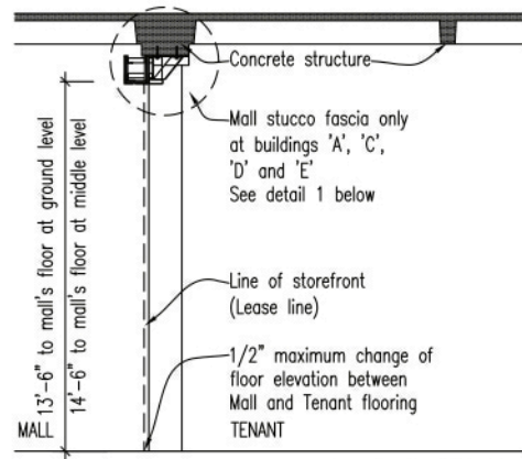
Longitudinal Section
